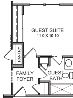
OPT. GUEST SUITE IN LIEU OF INC. CASUAL LIVING
